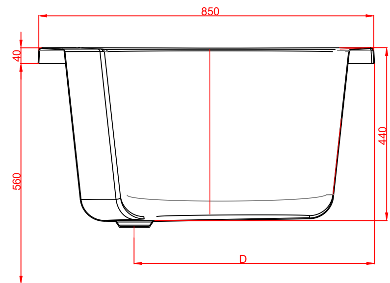
SECTION A-A SCALE 1:4
